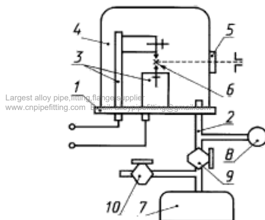
Рисунок Б.1 — Схема установки для выполнения анализов при пониженном давлении воздуха
